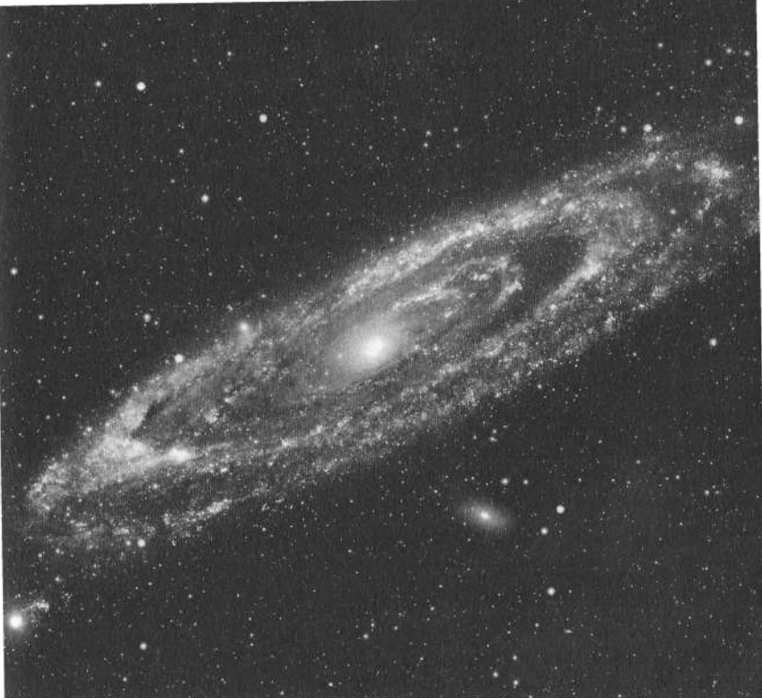
Andromeda Galaksisi
